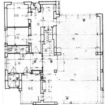
Grundriss Haus Ragip Bey 1:300
