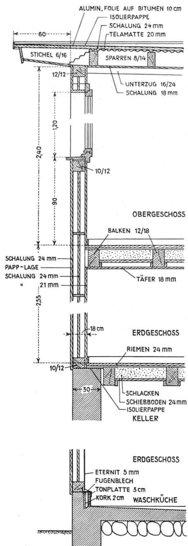
Konstruktionsdetail 1:40
