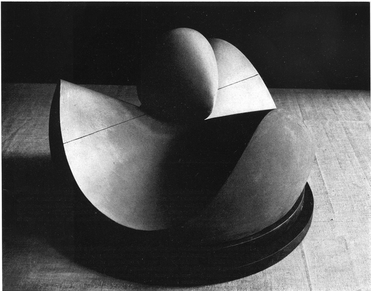
Mathematisches Modell von H. Henrici (1876), im Science Museum, London Darstellung der Formel xyz = k^2(x + y + z - 1)^2 (Aus «Moderne Plastik» von C. Giedion-Welcker)
