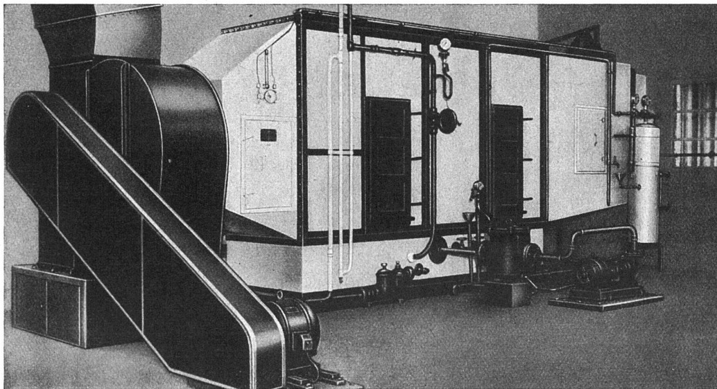
Ansicht einer Klima-Anlage (Ventilator, Luftwascher, automatische Regelapparate etc.), wie wir sie im Corso-Theater, Zürich, Kintheater Urban und Roxy, Zürich, Bei Air Metropole, Lausanne, etc. aufgestellt haben
