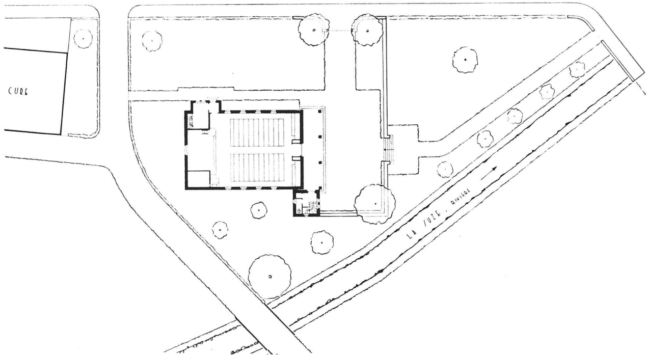
Eglise de Villeret Situation et plan 1:600, sections 1:400
