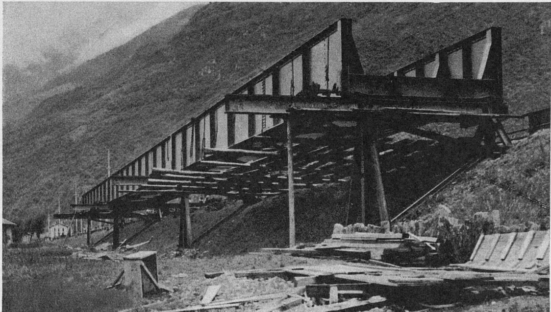
SBB eingleisige Bahnbrücke über die Moesa, Tessin Montage der Brücke auf Jochgerüsten neben dem Geleise
