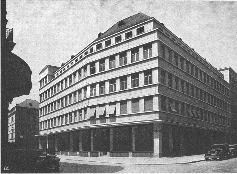
Geschäftshaus Schanzeneck Zürich, 1933 (Fortsetzung der Börse) Fassaden - Verklei- dung aus mehrfar- bigem, künstlichem Muschelkalk. Ge- sägt imitiert.
