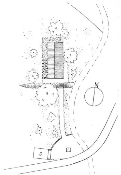
Situation 1:1000 / Plan de situation / Site
