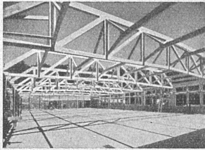
Vorfabrizierte Vorspannbeton-Konstruktion Vobag AG. Zürich
