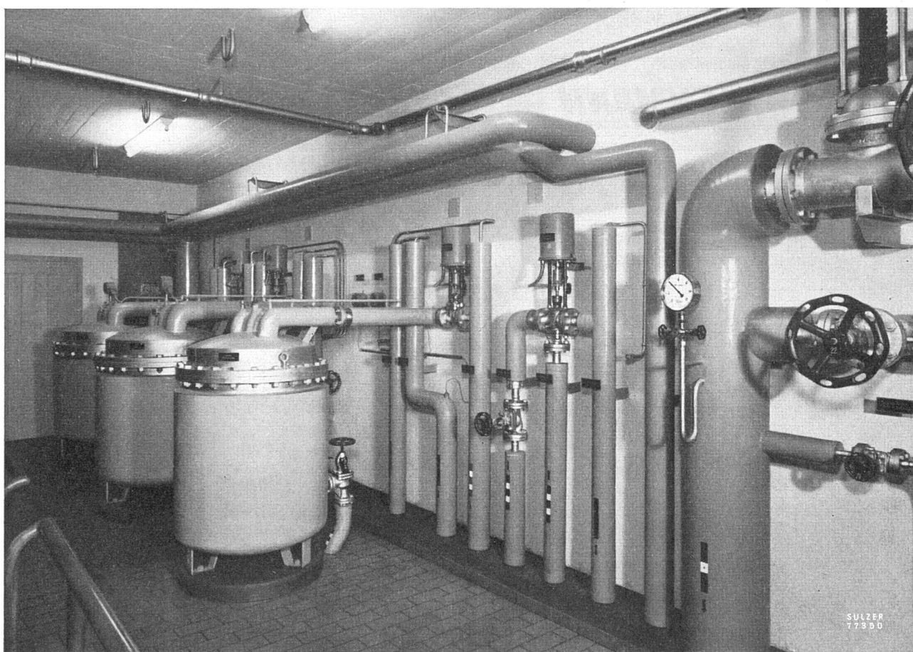
Ausschnitt aus dem Apparateraum - Umformer für Warmwasser-Bereitung und Raumheizung
