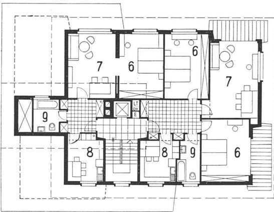
Neuntes Geschoß 1:300 | 9e étage | 9th upper floor
