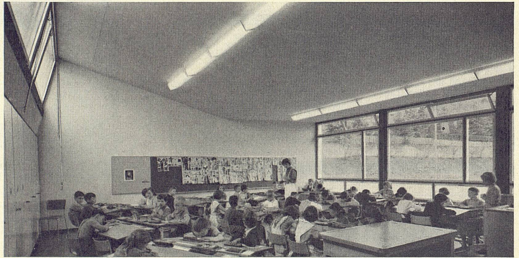
➔ Ausgleich der Oberlicht- verluste durch Konvek- torstreifen
