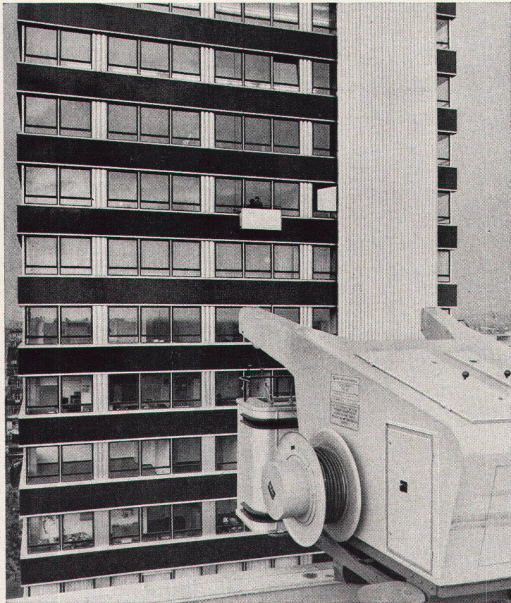
Phoenix-Rheinrohr AG Thysenhaus Düsseldorf Außenbefahreinrichtung
