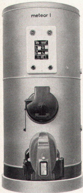
meteor I Kombiheizkessel mit grosser Leistung. Umstellbar von Oel auf feste Brennstoffe.
