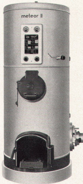
meteor II Doppelbrand-Kombiheizkessel mit 2 getrennten Brennkammern. Kann gleichzeitig mit Oel auch andere brennbare Stoffe verfeuern.
