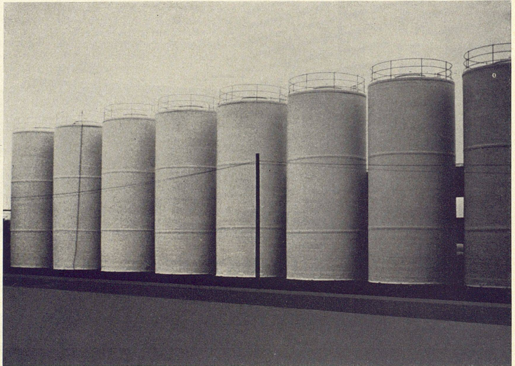
Centre Agricoles, Geigy, St-Aubin – 8 MWB-Gärfuttersilos zu je 200 m 3
