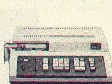
CS 662 16 Stellen. Ein Rechenpeicher. Ausgerü- stet mit neuartigem chemischem Schreiber, der in Sekundenbruchteilen 16stellige Werte lautlos auf horizontalem Papier- streifen in Klarschrift wiedergibt. 34,6 x 12,7 x 42,8 cm. 8 kg. Fr. 4250.-
