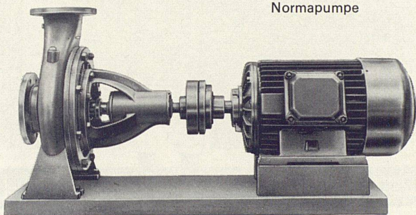
Normpumpe
