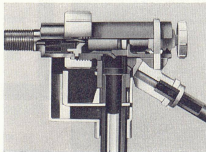
Neues GEBERIT-Schwimmventil Modell 1970.
