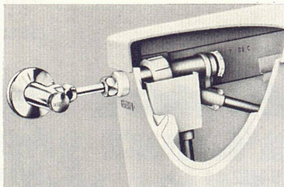
Die bewährte GEBERIT-Vollisolation gegen Schwitzwasserbildung.
