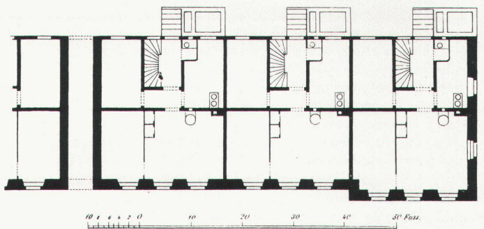
Grundriss Erdgeschoss einer Häuserreihe 1861
