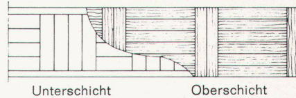
Schnittbild einer Parkettziele
