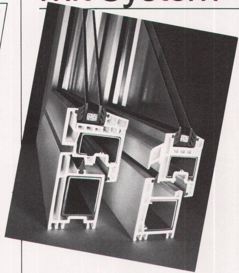
2flügliges Dreh-/Kippfenster ohne Setztstück
