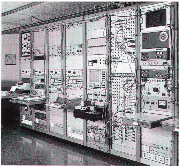
Luftschallprüfung EMPA Zürich
