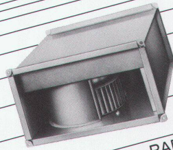
Kanalventilatoren
