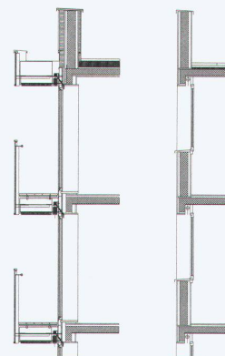
Fassadenschnitt neu
