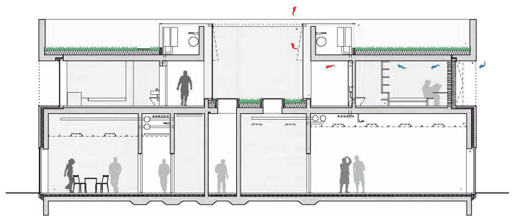
Konstruktionsschnitt durch Wohn- und Arbeitsgeschoss
