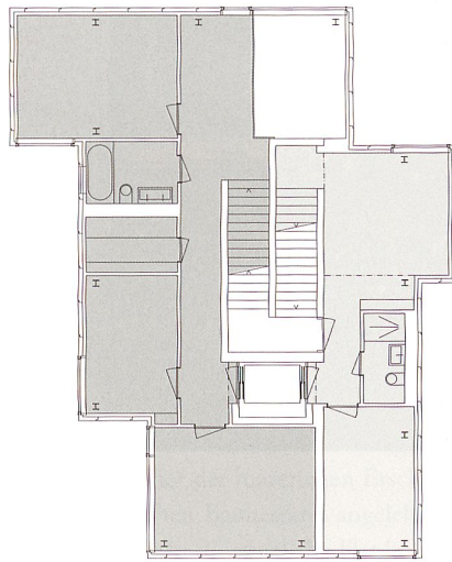
1. Obergeschoss
