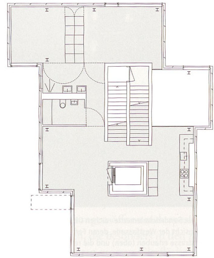
2. Obergeschoss
