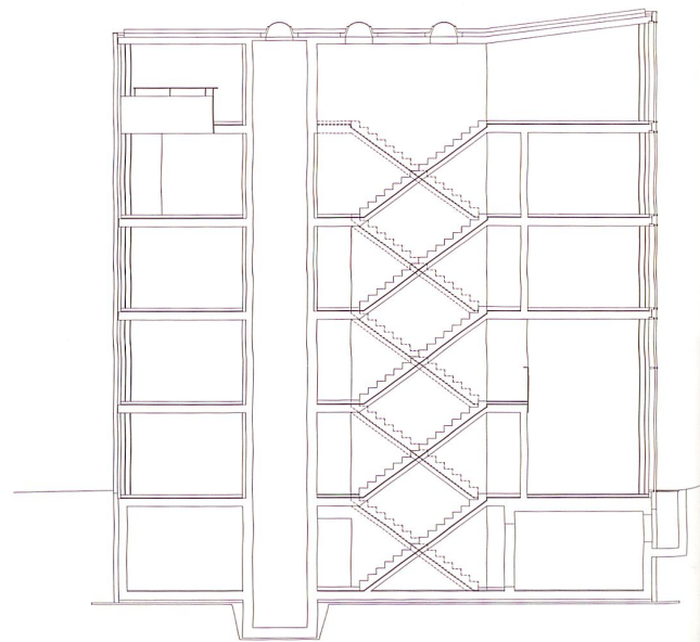
Längsschnitt
