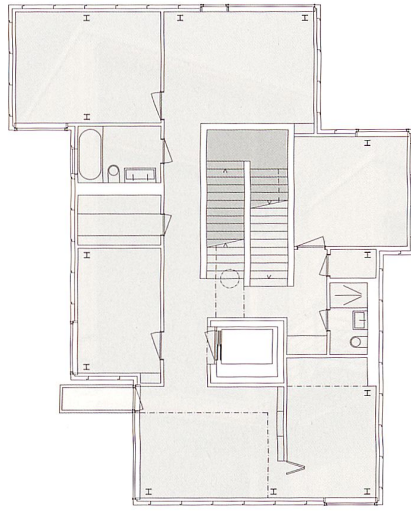
3. Obergeschoss
