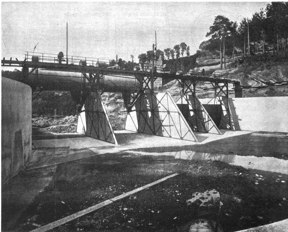
Abbildung 3. Segmentschützwehr in Thusy-Hauterive (Freiburg).
