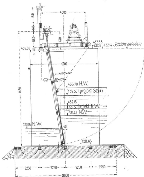
Abb. 5. Die Vergrößerung des Niederwasserabflusses aus den Juraseen. Das Nidauerwehr nach dem Umbau. Querschnitt durch die linksseitigen Mittelschützen. 1 : 200.
