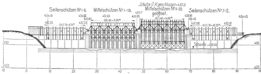
Abb. 4. Die Vergrößerung des Niederwasserabflusses aus den Juraseen. Das Nidauerwehr nach dem Umbau. Ansicht von 3 m oberhalb den Schützen. 1 : 800.
