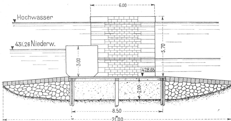
Abb. 2. Die Vergrösserung des Niederwasserabflusses aus den Juraseen. Das Nidauerwehr vor dem Umbau. Querschnitt durch die Mittelöffnung. 1 : 200.
