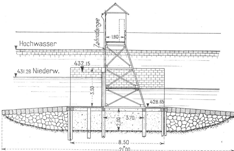
Abb. 3. Die Vergrösserung des Niederwasserabflusses aus den Juraseen. Das Nidauerwehr vor dem Umbau. Querschnitt durch die Seitenöffnung. 1 : 200.
