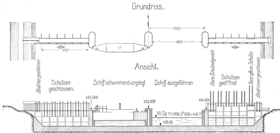
Abb. 1. Die Vergrösserung des Niederwasserabflusses aus den Juraseen. Das Nidauerwehr vor dem Umbau. Ansicht und Grundriss. 1 : 800.
