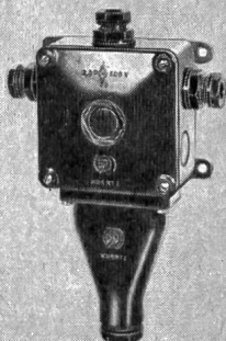
Bakelitdose mit angebautem, druckfestem Endverschluss
