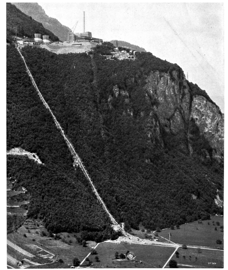
Fig. 3 — Vue aérienne de la centrale de Vouvry, montrant sa position surélevée à environ 450 m au-dessus du fond de la vallée, choisie pour éviter tout danger de pollution de l'air. Le combustible provenant de la raffinerie voisine y est chauffé à 120°C pour être pompé, ainsi que l'eau d'appoint, de la vallée à la centrale.
