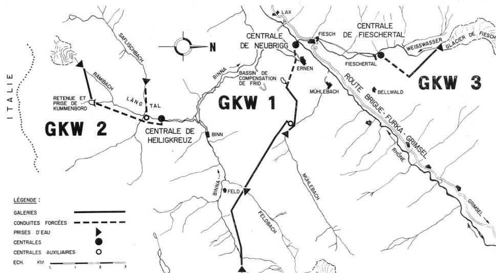
Fig. 2 Aménagement des Forces Motrices de Conches S.A.; Conception complète.
