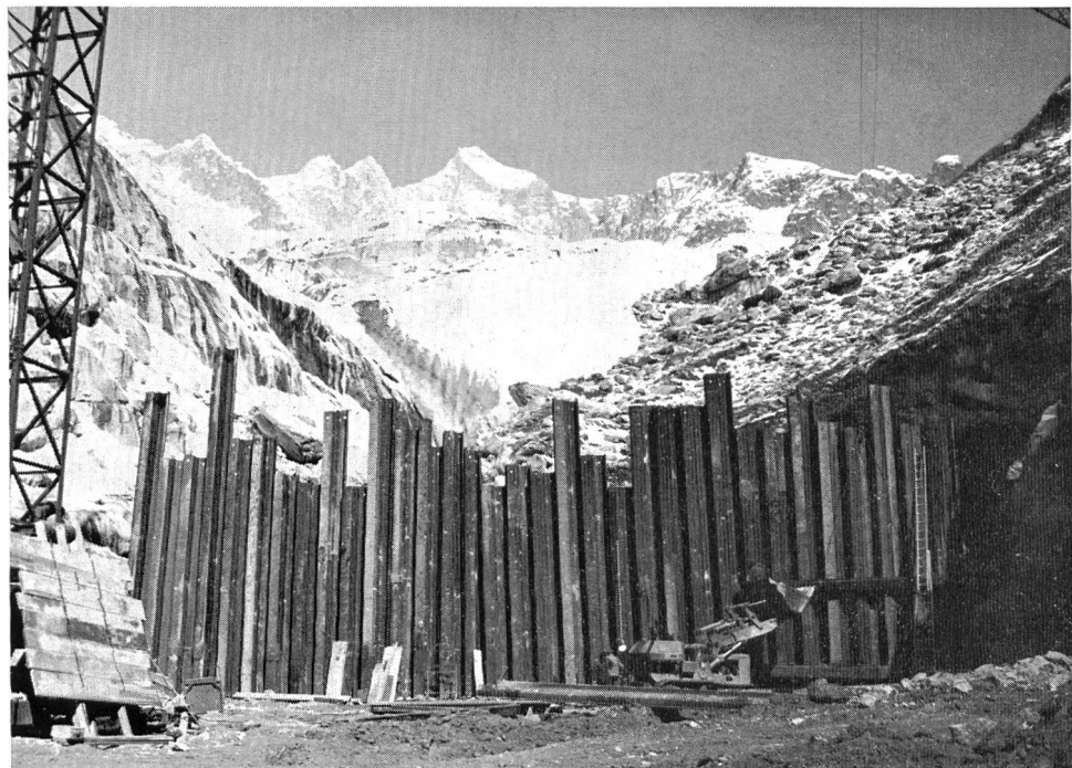
Fig. 1 Forces Motrices de Conches S.A./Gommerkraftwerke AG: GWK III Chantier de la prise d'eau près du glacier de Fiesch; rideau de palplanches.
