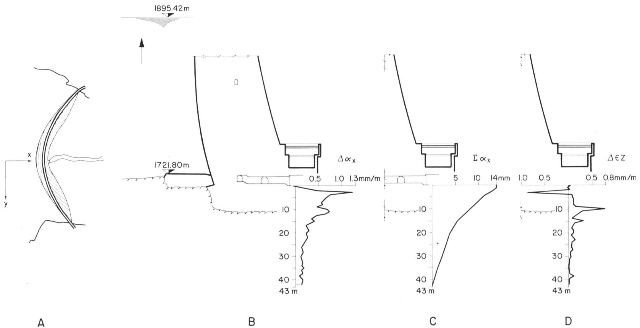
Figure 6. Kölnbrein, barrage-voûte, bloc 17. Trivec, résultats des mesures pour remplissage. A Vue en plan avec x et y axes B Développement des déformations horizontales différentielles \alpha_x C Développement des déformations horizontales \Sigma \alpha_x D Développement des déformations différentielles verticales \epsilon_z
