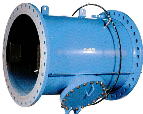
Ausbaurohr Tubo di rivestimento Tuyau de démontage
