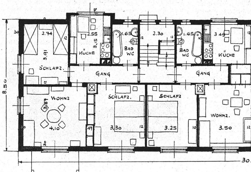
Gemeinnützige Bau- und Wohngenossenschaft „Freistatt“, Thun Wohnungsgrundriß
