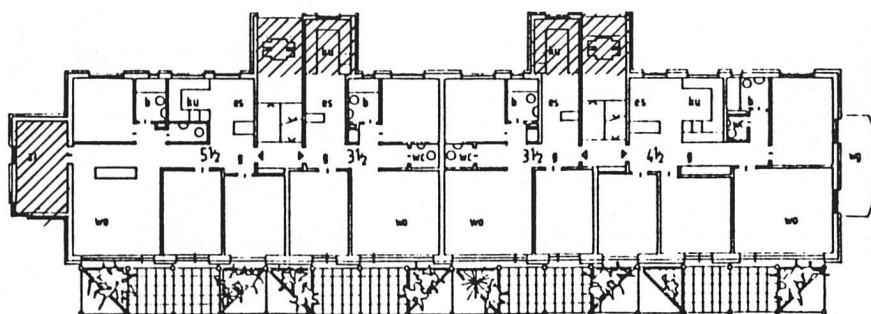
Stufe 3: Umbau/Neubau von Fassade, Balkon-/Pflanzengerüst, Wintergarten, erweiterten Küchen-Essplätzen, Schlafzimmer, separatem WC, erweitertem Treppodest als «Nachbarschafts-Kollektivzone».
