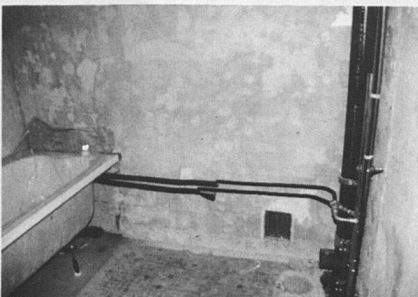
Montage der Steig- und Fallstränge.
