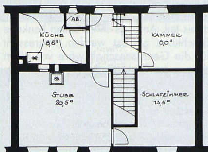
Grundriss einer Obergeschoss-Wohnung Wohnzimmer in der Fuggerei
