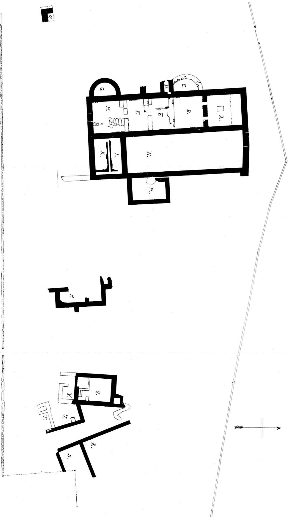
Fig. 50. Grundriß der röm. Fundamente in der Curstorei in Chur.
