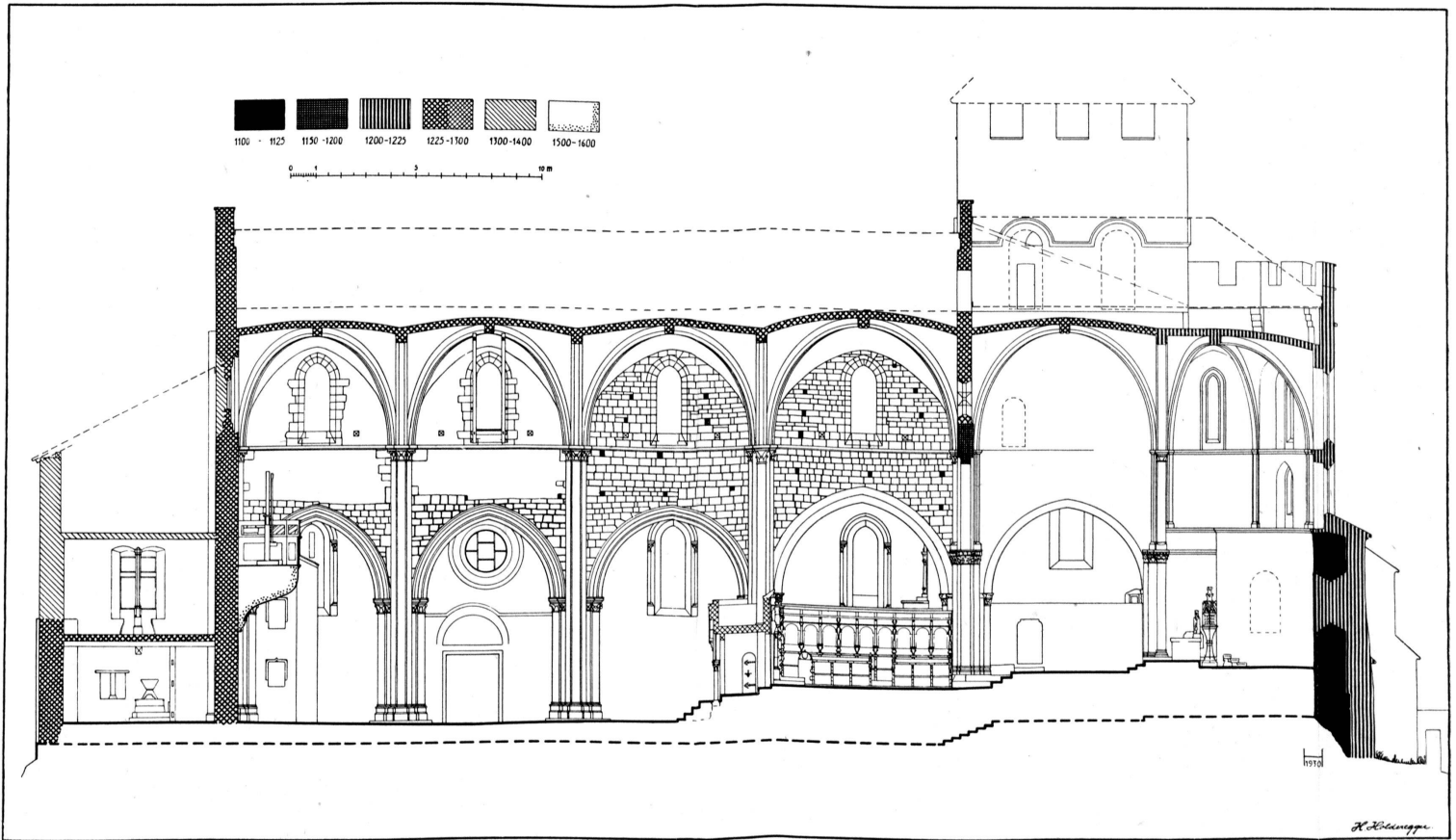
Die Kirche von Valeria. Längsschnitt 1 : 200.
