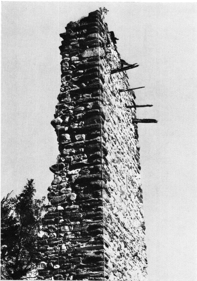
Abb. 3 Cagliatscha (GR). Markante Bossenquader im Eckverband
