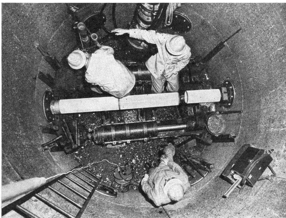
Einbau der Kunststoff- filterrohre im Schacht eines horizontalen Filterbrunnens
