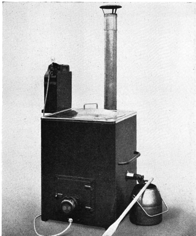
Kochkessel 150 Liter mit Isosem Deckel. Feuerung mit flüssigen oder festen Brennstoffen. ▼▼
