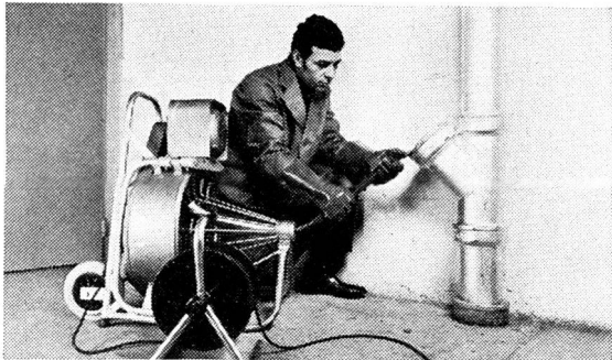
Entstopfer Typ A20 für Rohre von 50–300 mm \varnothing und bis zu 30 m Länge. Für Rohre über 300 mm \varnothing lohnt sich der Einsatz unserer «Atümat»-Hochdruckreinigungsgeräte.
