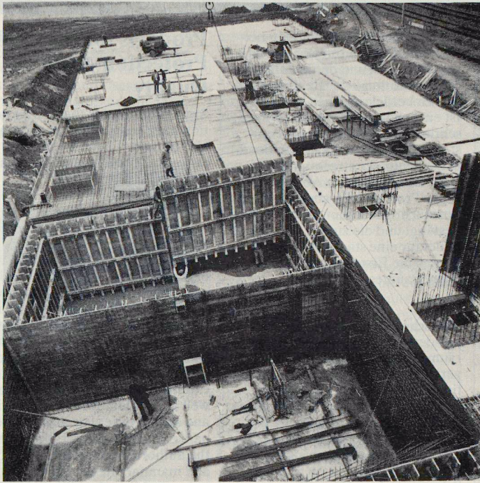
John's Oil AG, Cham: 8 Betontanks zur Lagerung von Heiz- und Dieselöl mit einem Totalinhalt von 5 Millionen Litern. Auskleidung: BORSAFOIL-Polyester-Doppelmantel.
