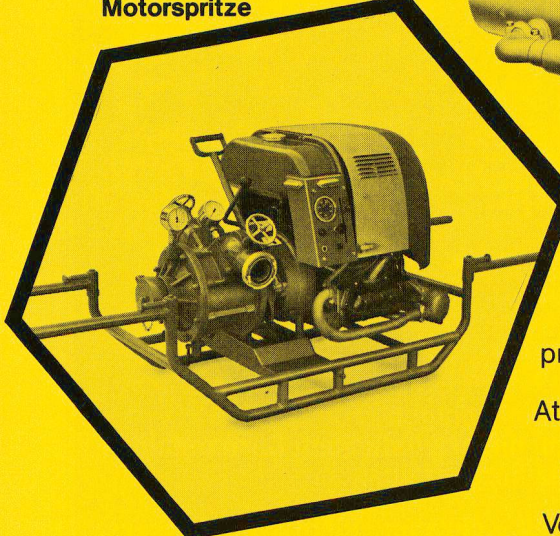
Motorspritze
