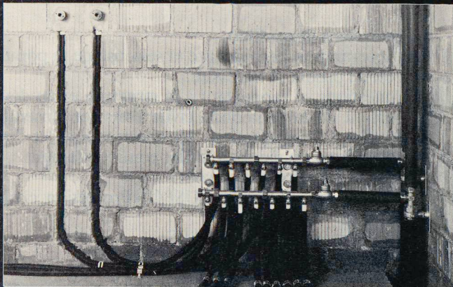
SANIPEX-System JRG® ist eine «Rohr in Rohr-Installation»
