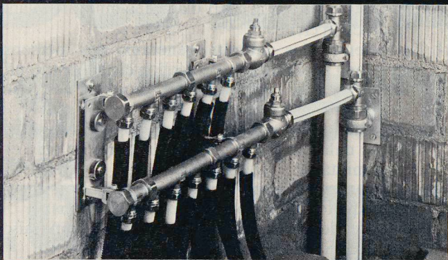
SANIPEX-System JRG® spart Montagekosten durch Wegfall aufwendiger Arbeitsvorgänge
