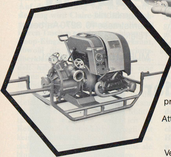
Motorspritze
