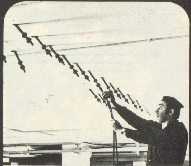
Wassereinbrüche – Abdichtung mit Renesco-Flexin-Injektionen
