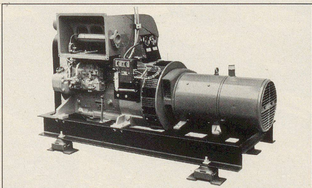
Notstromanlagen. NEMP geschützt, schocksicher installiert, mit BZS-Zulassung. Leistungsbereich 20 – 150 kVA.
