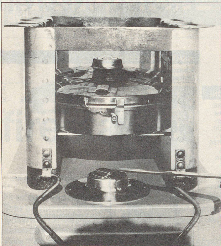
2 Firestar-Sicherheitsbrenner in Rost eingesetzt 2 brûleurs de sécurité Firestar en position dans le foyer d'autocuiseur 2 elementi di combustione Firestar posti nella griglia
